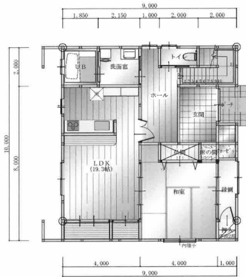
1階 平面図 S:1/80
