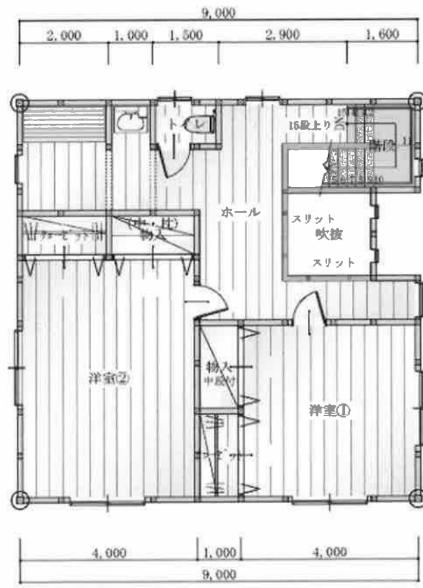
2階 平面図 S:1/80
